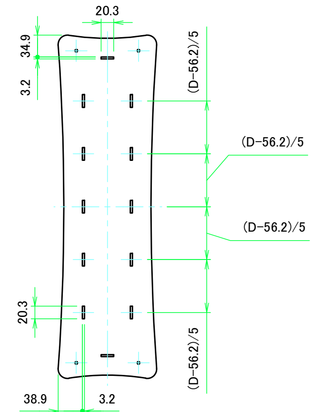
上カバー裏面 / Top cover Backside
