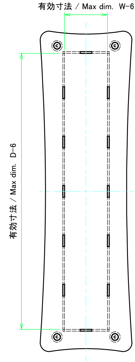
下カバー / Bottom cover
